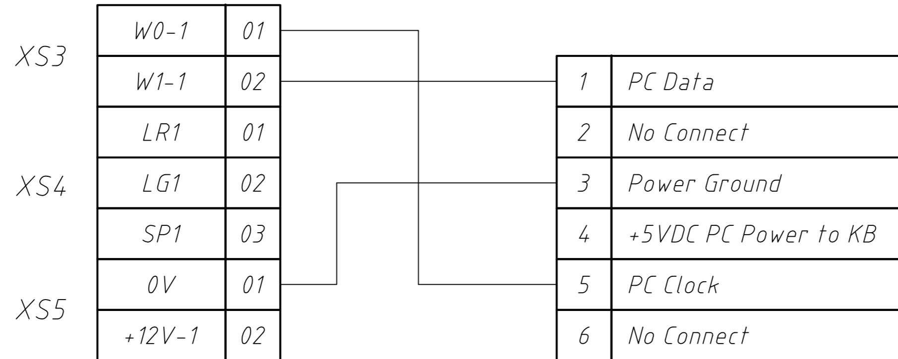
Контакты контроллера ACS-105-CE
